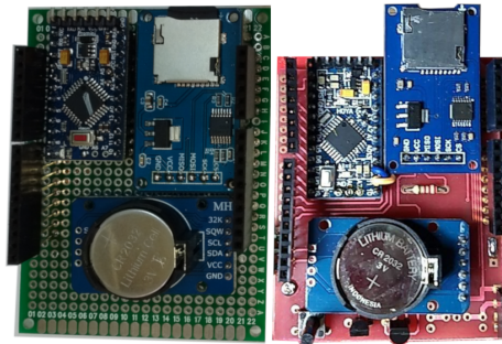
Figura 1. Datalogger, sobre protoboard (izq.) y montado en PCB (der.).
