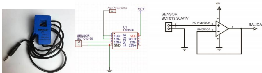
Fig. 4. Sensor de Corriente SCT-013-000 y Circuito de conexión del sensor SCT-013-000 y el operacional LM358
